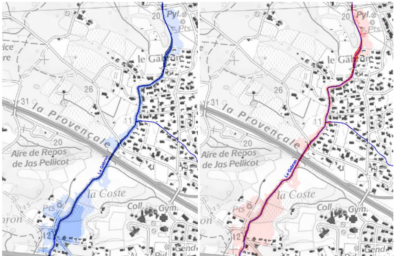
Figure 24 : Hauteur d'eau et vitesses d'écoulement – Le Gabron
