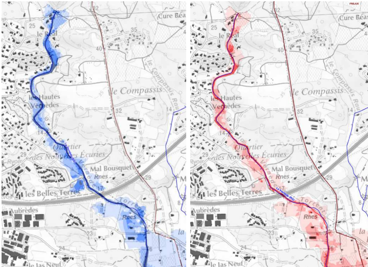
Figure 25 : Hauteur d'eau et vitesses d'écoulement – La Vernède
