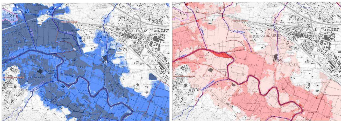
Figure 23 : Hauteur d'eau et vitesses d'écoulement – L'Argens
