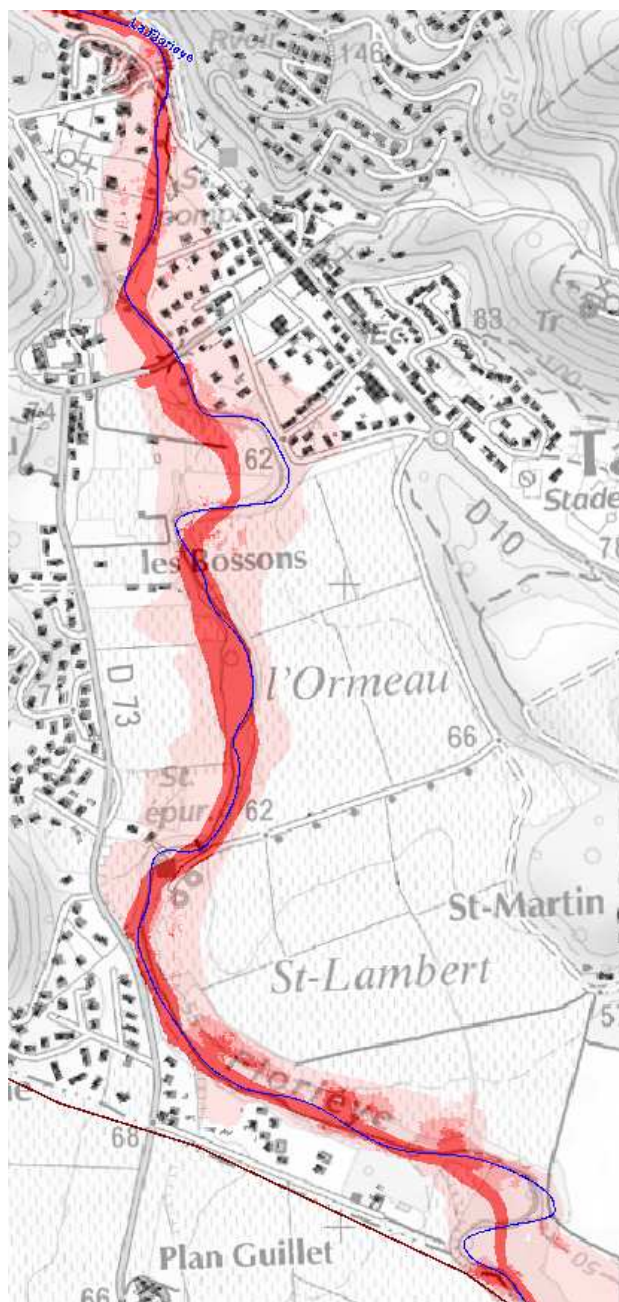
Figure 24: Hauteurs d'eau et vitesses d'écoulement : Rives urbanisées de la Florieye
