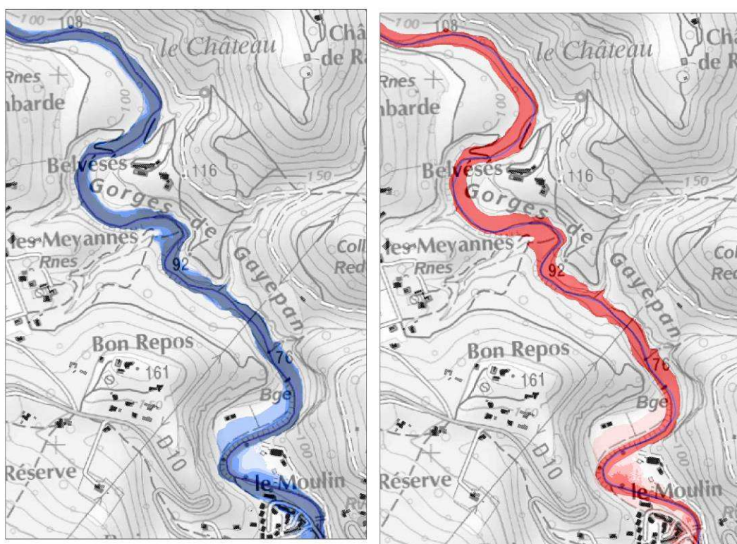
Figure 23: Hauteurs d'eau et vitesses d'écoulement : Gorges de la Florieye
