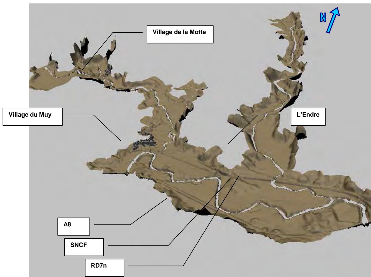
Vue globale du modèle de la Nartuby aval
