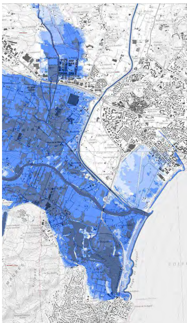
Hauteur d'eau et vitesses d'écoulement – L'Argens
