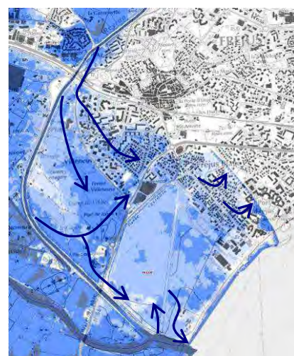
Effacement des digues avec Crue de référence Argens ou crue de référence Reyran
