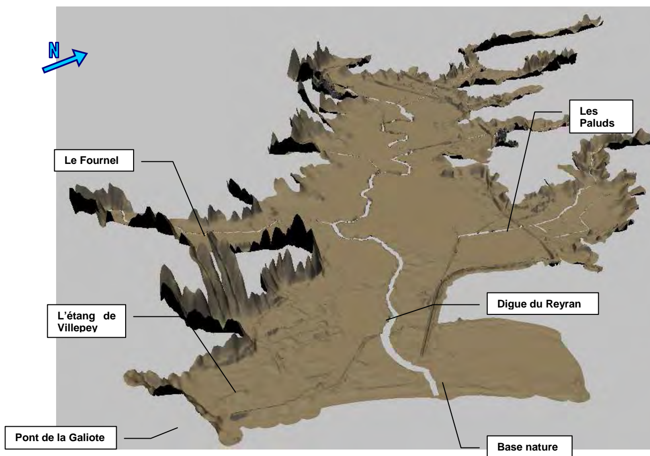
Vue globale du modèle de la basse plaine de l'Argens
