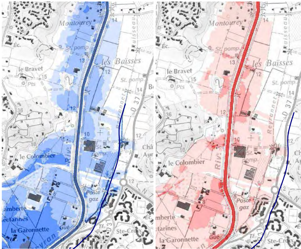
Hauteur d'eau et vitesses d'écoulement
