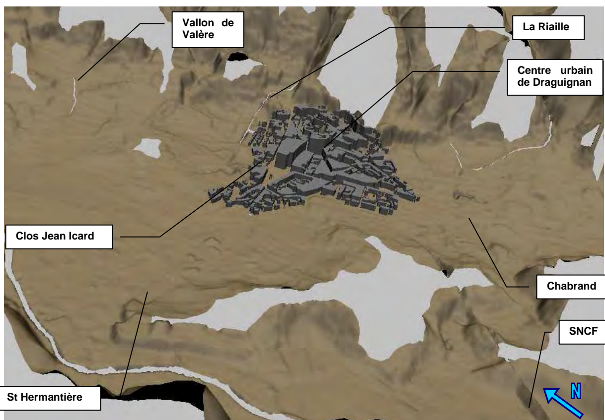
Vue du modèle de la Nartuby à Draguignan au niveau du centre urbain de Draguignan
