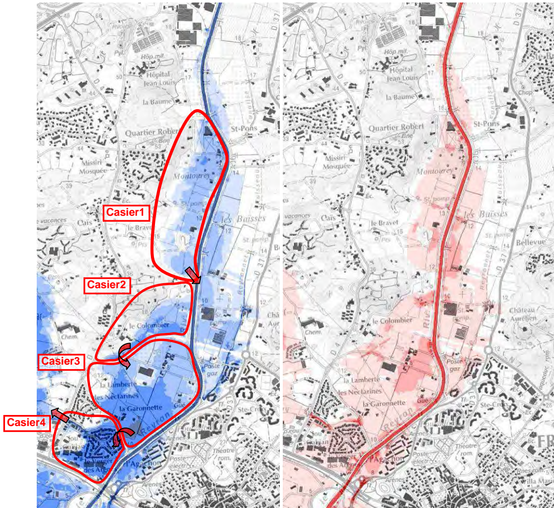
Hauteur d'eau et vitesses d'écoulement –Rive droite de la plaine du Reyran
