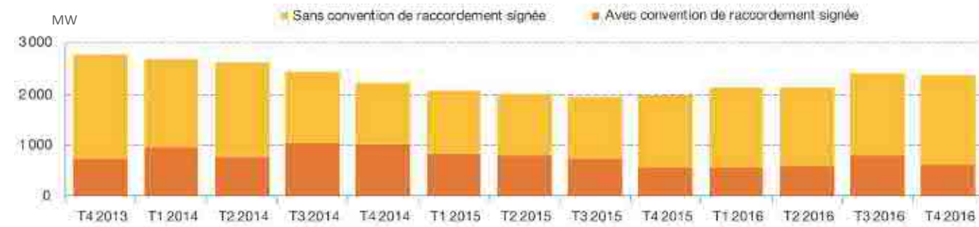
Evolution de la puissance des projets solaires photovoltaïques en cours d'instruction (source : SOeS d'après Enedis, RTE, EDF-SEI et les principales ELD)
