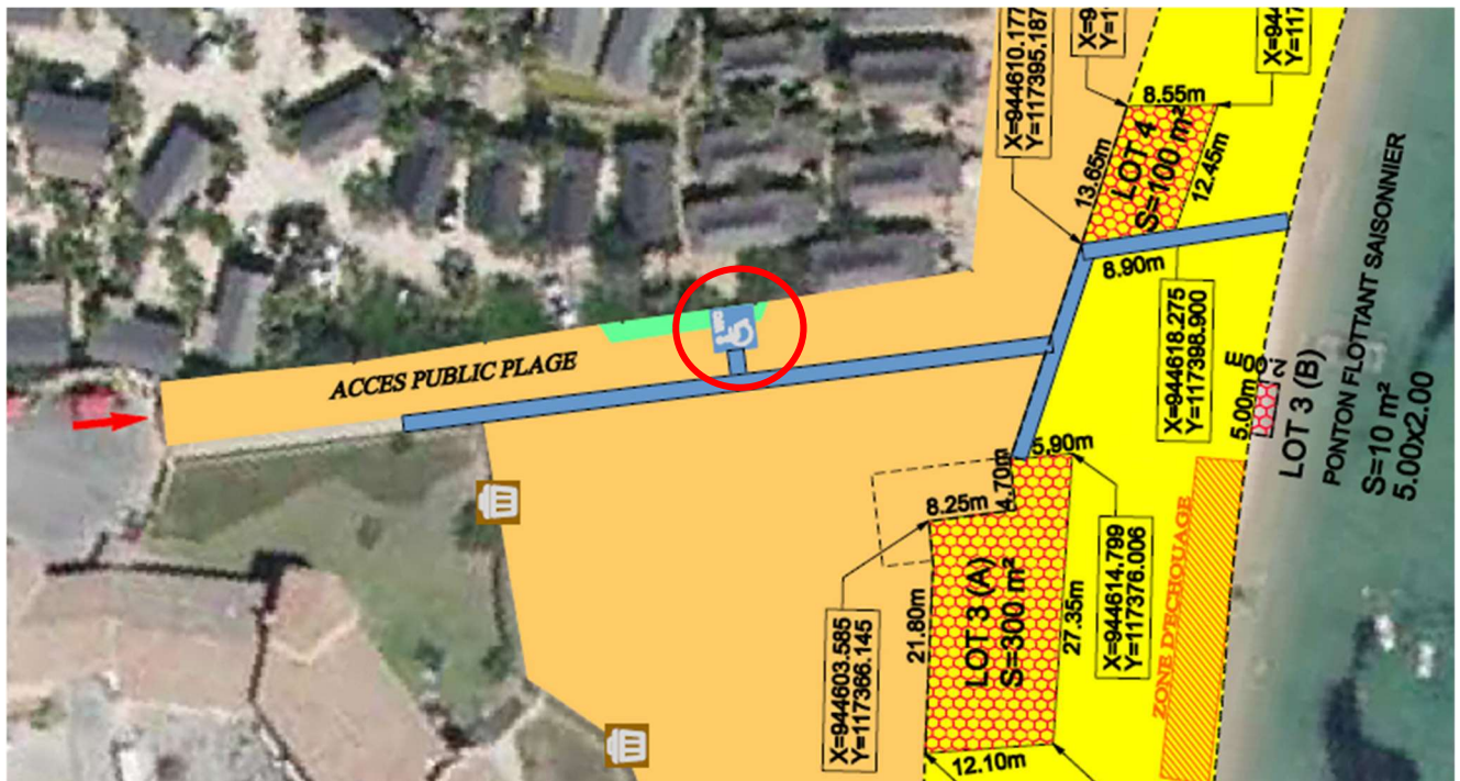
Figure 14 - Extrait du plan de concession projetée, illustrant la position des sanitaires accessibles PMR et leur desserte par le platelage bois communal
