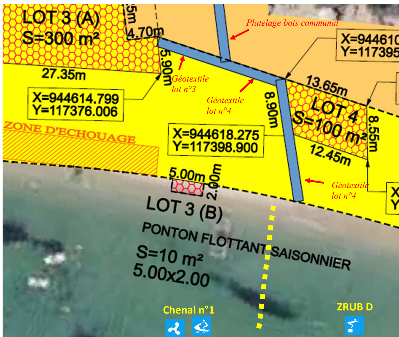
Figure 8 -Extrait du plan de concession projetée, illustrant la desserte du plan d'eau par le tapis en géotextile (en bleu)
