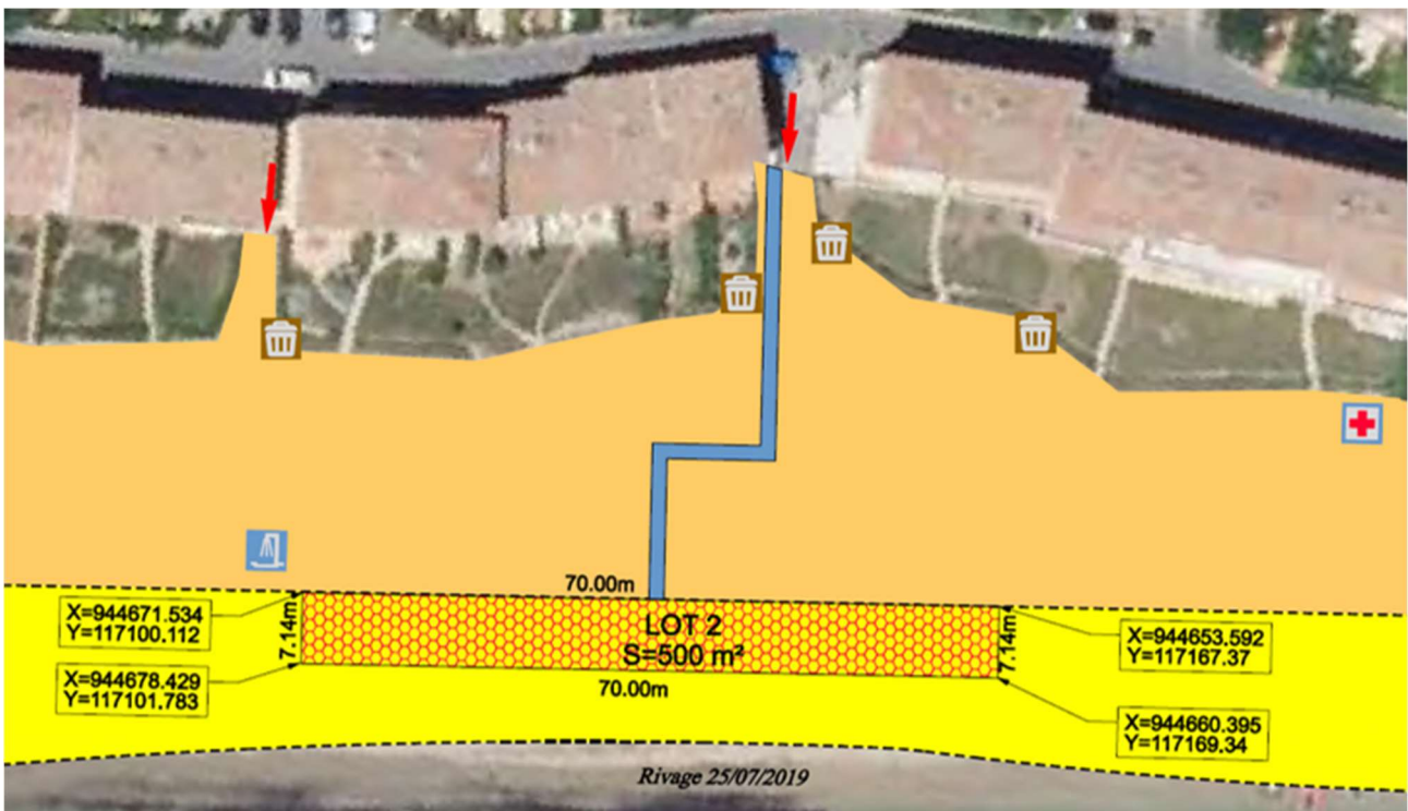
Figure 9 - Extrait du plan de concession projetée, illustrant la desserte du lot de plage par le tapis en géotextile (en bleu)
