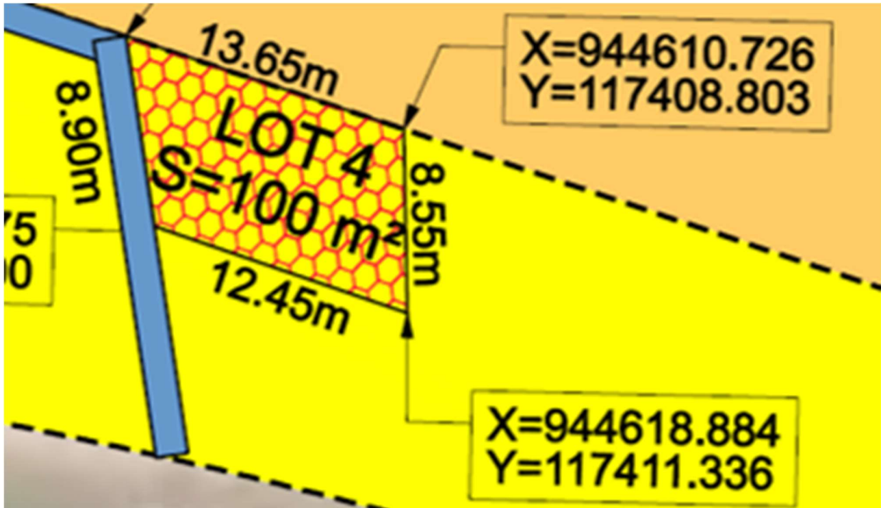
Figure 13 - Extrait du plan de concession projetée, illustrant la desserte du lot de plage par le tapis en géotextile (en bleu)
