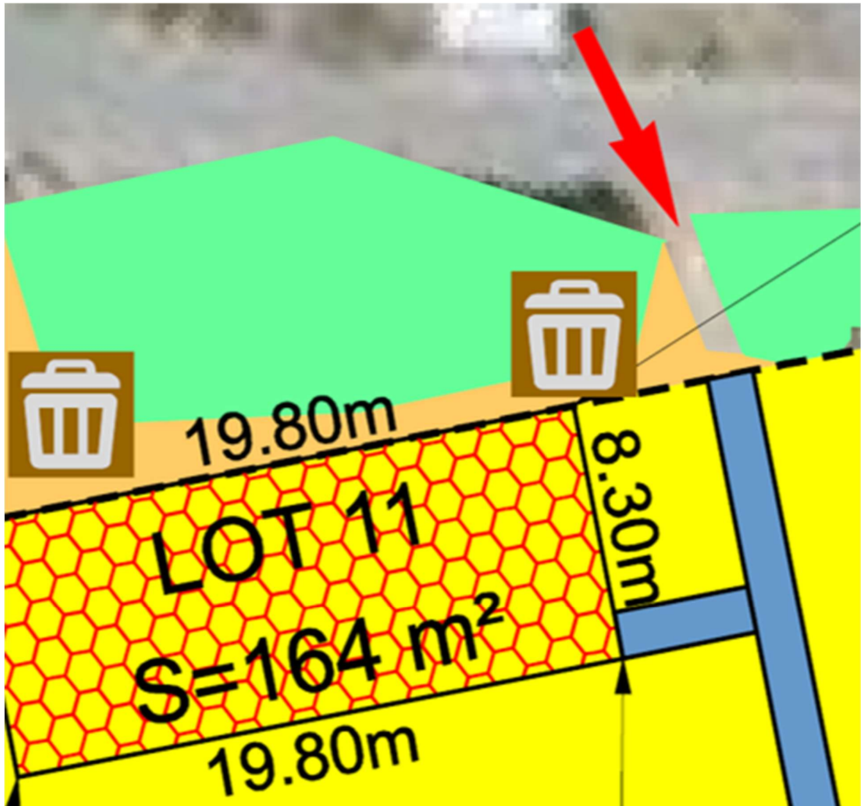
Figure 11 - Extrait du plan de concession projetée, illustrant l'accès au lot de plage par le tapis en géotextile (en bleu)
