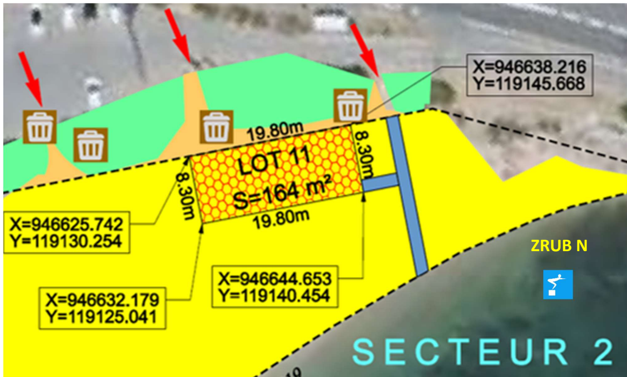
Figure 10 - Extrait du plan de concession projetée, illustrant l'accès au plan d'eau par le tapis en géotextile (en bleu)
